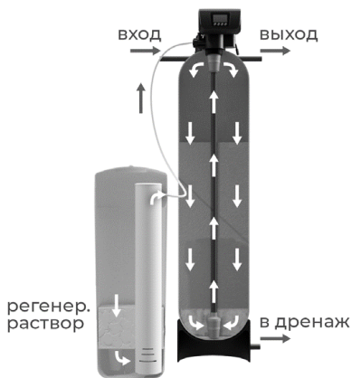
2. Подача реагента
